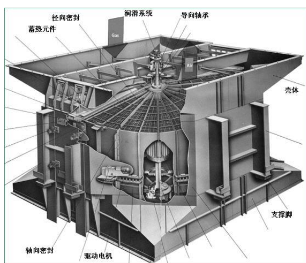
空气预热器结构示意图
