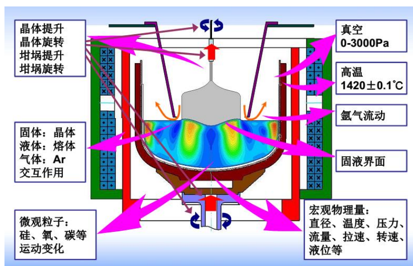
硅单晶炉工作环境示意图
