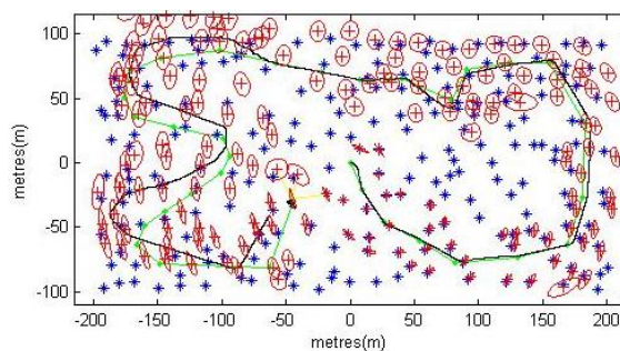
估计的 3\sigma 区域图
