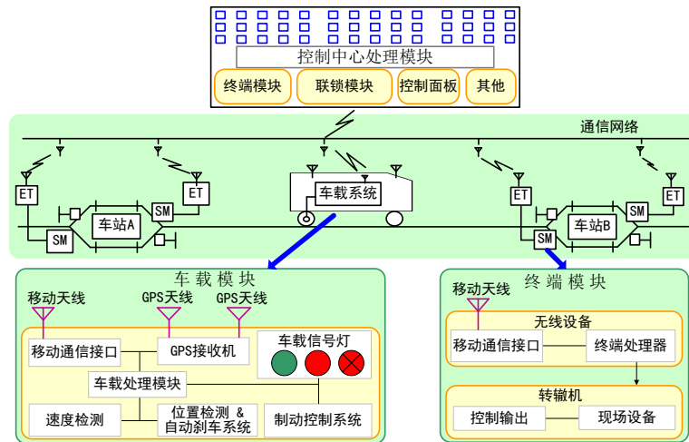
列车控制系统结构图
