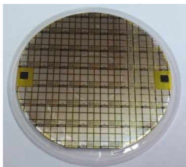
SiC 晶圆片
