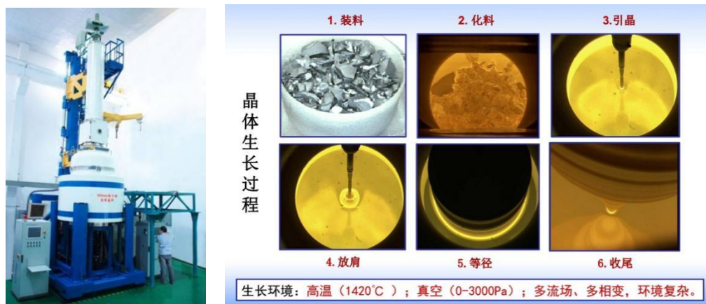
电子级硅单晶炉
